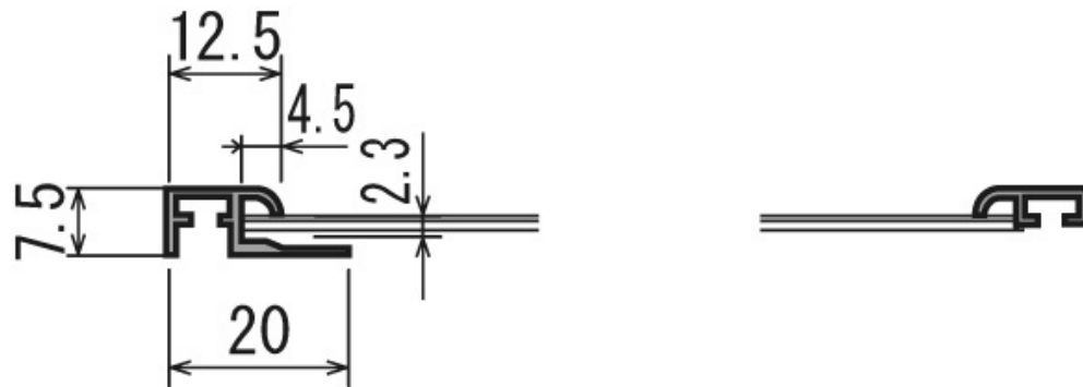
フレーム断面図
