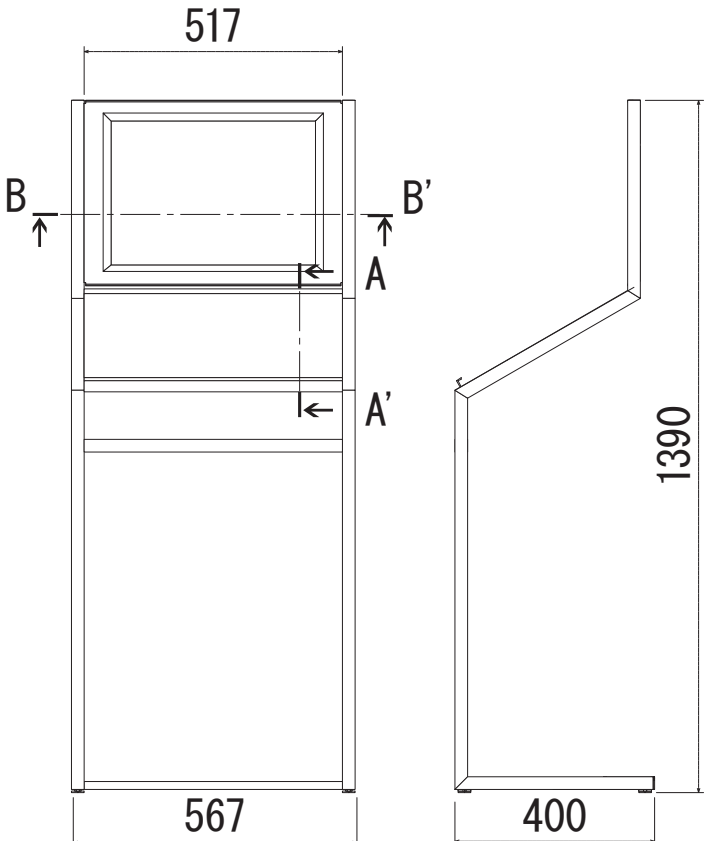
寸法図
